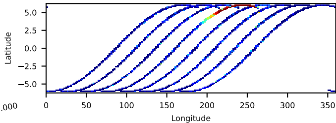
80202006004: 30 to 120 keV
