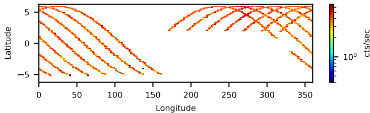
80102002006: 3 to 120 keV
