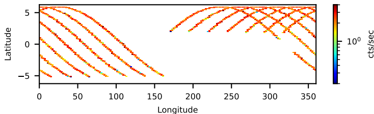
80102002006: 3 to 10 keV
