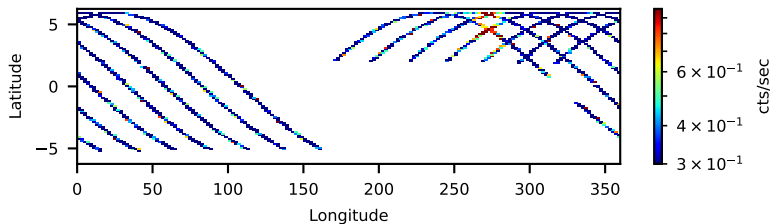
80102002006: 30 to 120 keV
