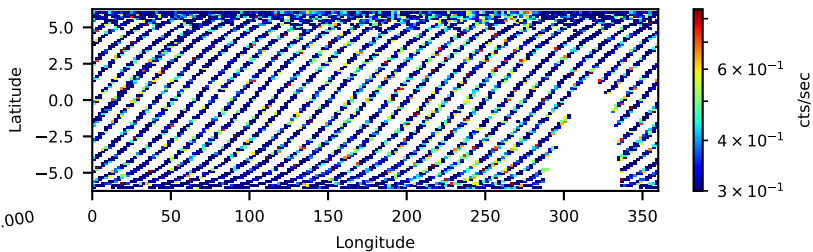
80002096004: 30 to 120 keV
