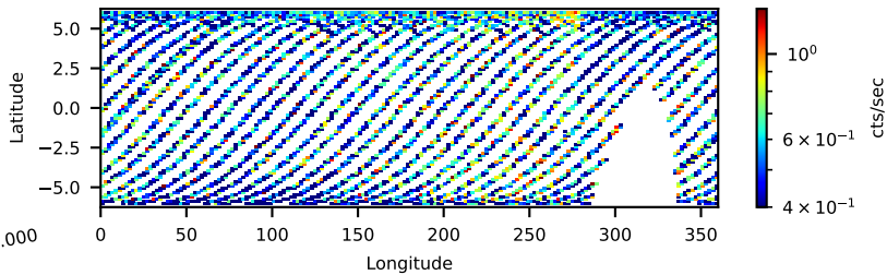
80002096004: 3 to 10 keV
