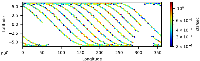
80001002004: 30 to 120 keV
