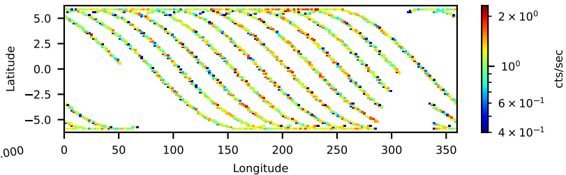
80001002004: 3 to 10 keV
