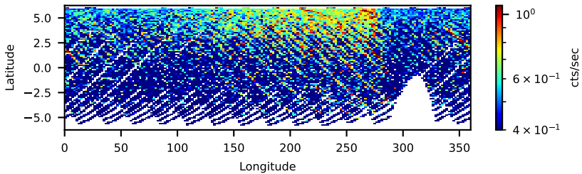
70901004002: 3 to 120 keV
