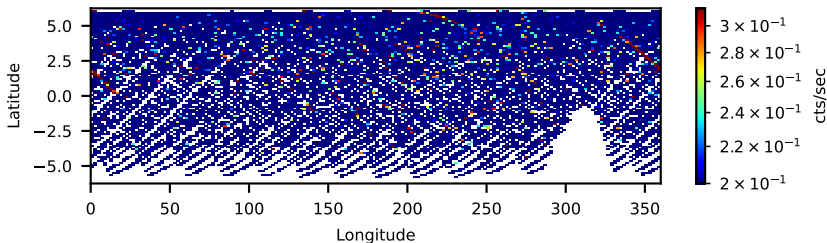
70901004002: 3 to 10 keV
