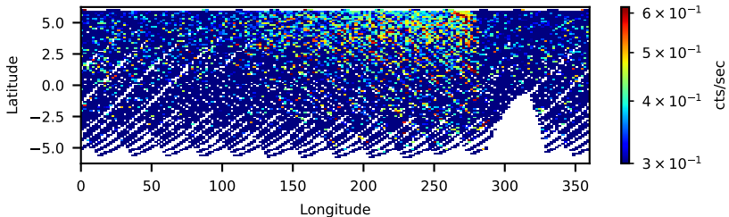
70901004002: 30 to 120 keV
