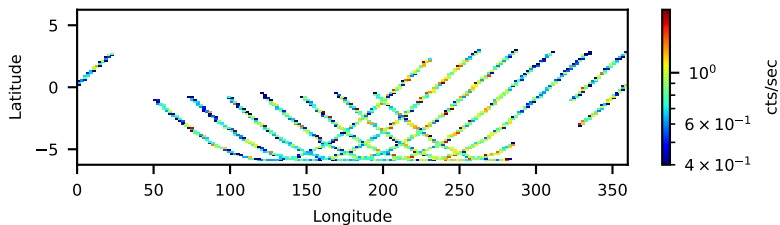
70860004002: 3 to 120 keV
