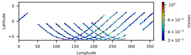
70860004002: 30 to 120 keV
