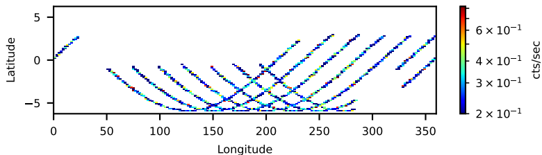
70860004002: 3 to 10 keV
