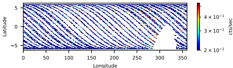
70102001002: 3 to 10 keV
