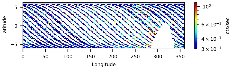
70102001002: 30 to 120 keV
