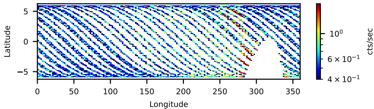
70102001002: 3 to 120 keV
