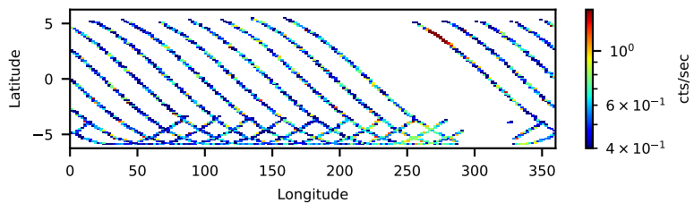
61064003002: 3 to 120 keV
