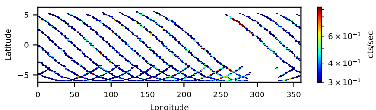
61064003002: 30 to 120 keV
