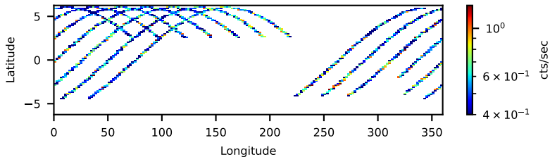
61063005002: 3 to 120 keV
