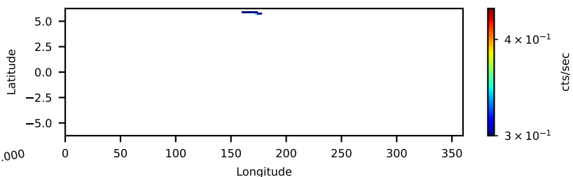
61060001001: 30 to 120 keV
