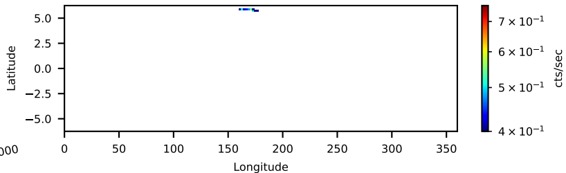
61060001001: 3 to 10 keV
