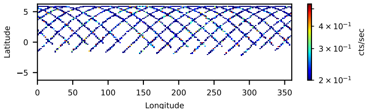
61002022006: 3 to 10 keV
