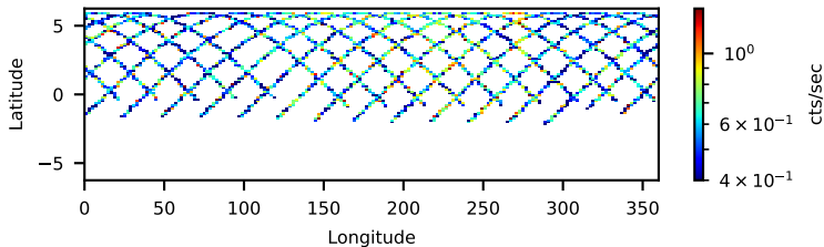
61002022006: 3 to 120 keV
