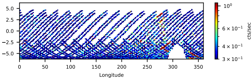
61002011006: 30 to 120 keV
