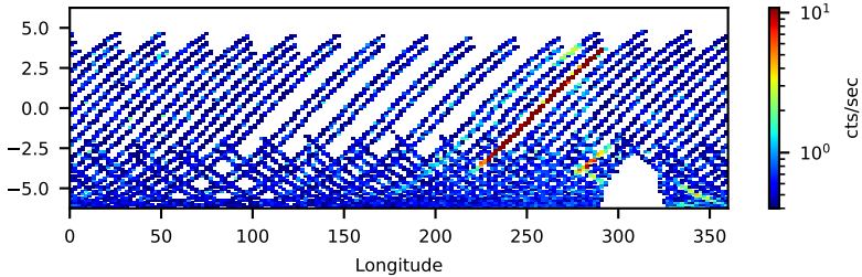
61002011006: 3 to 10 keV
