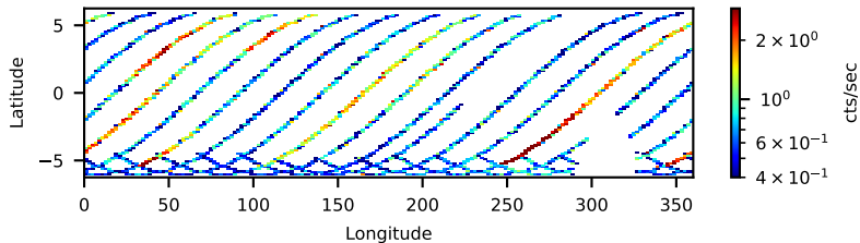
61002005002: 3 to 120 keV
