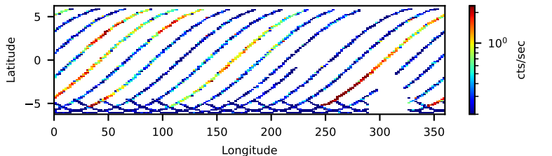
61002005002: 3 to 10 keV
