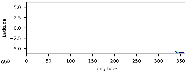
61001036001: 3 to 10 keV
