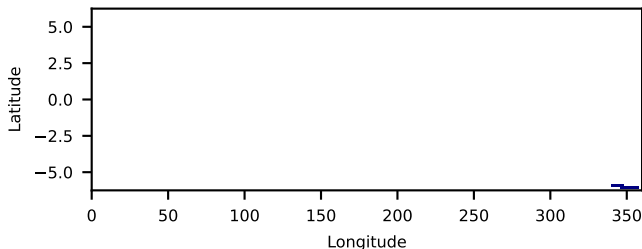
61001036001: 30 to 120 keV
