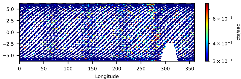
61001029002: 30 to 120 keV
