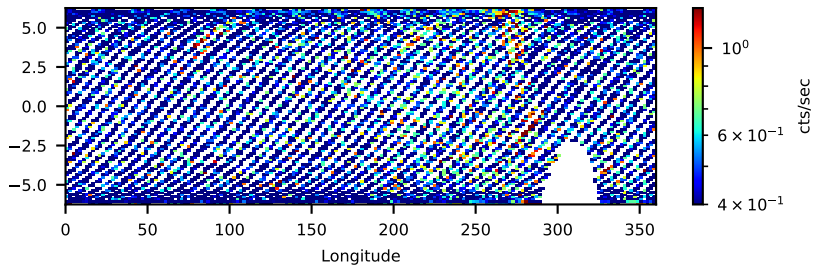
61001029002: 3 to 10 keV
