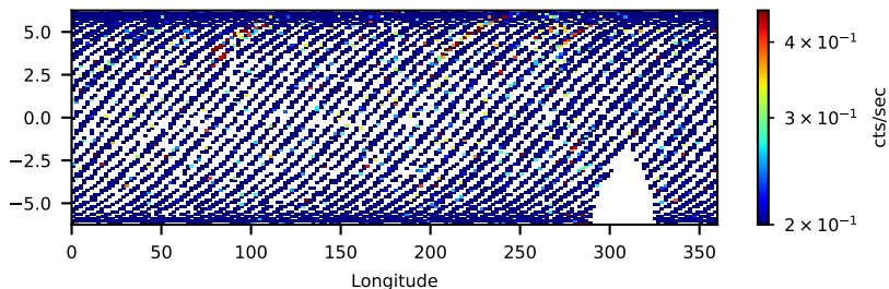
61001029002: 30 to 120 keV
