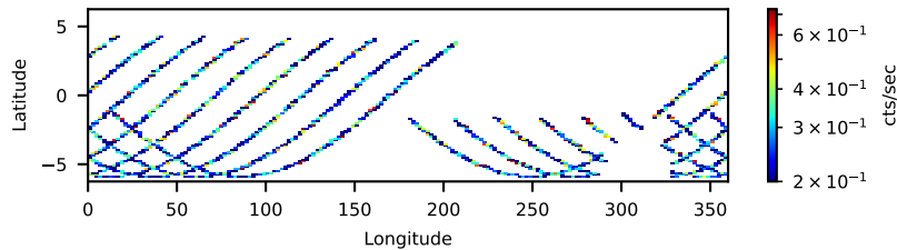
61001014002: 3 to 10 keV
