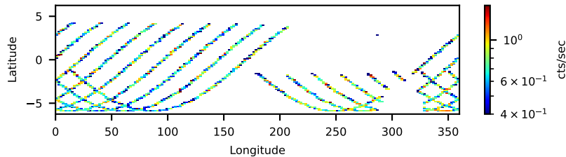
61001014002: 3 to 120 keV
