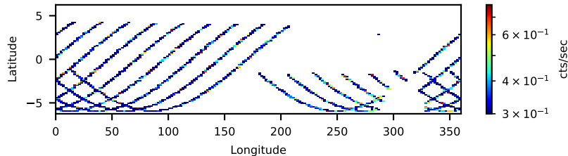
61001014002: 30 to 120 keV
