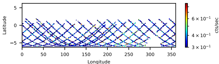
61001007004: 30 to 120 keV
