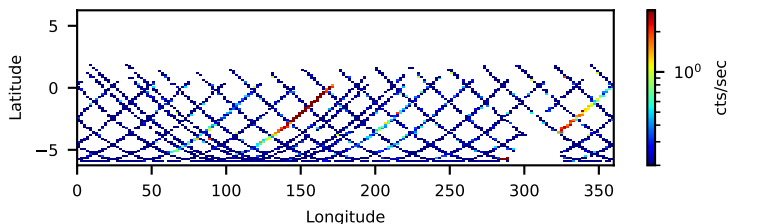
61001007004: 3 to 10 keV
