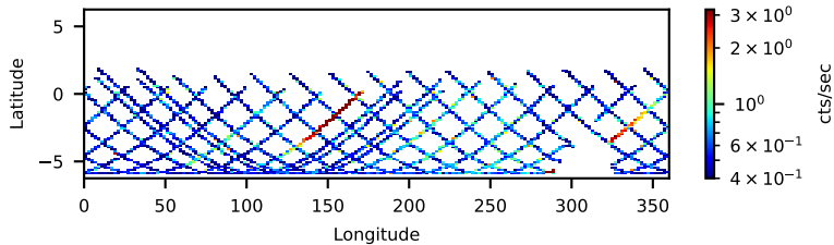
61001007004: 3 to 120 keV
