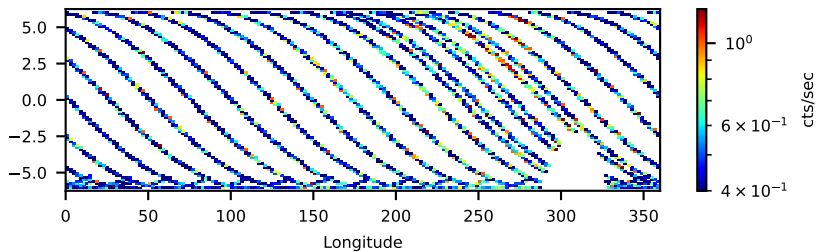
61001004004: 3 to 10 keV
