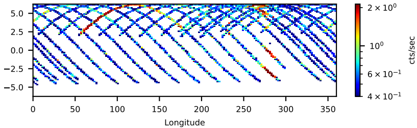
61001004002: 3 to 10 keV
