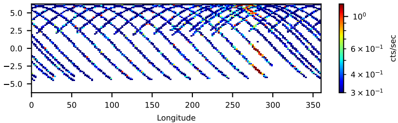
61001004002: 30 to 120 keV
