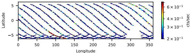
60965005003: 3 to 10 keV
