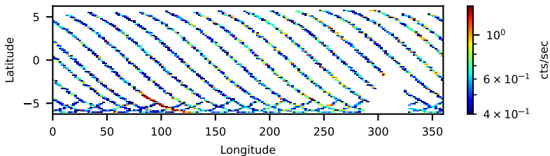
60965005003: 3 to 120 keV
