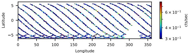
60965005003: 30 to 120 keV
