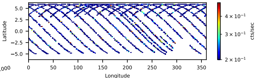
60965001002: 30 to 120 keV
