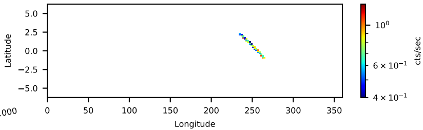
60965001001: 3 to 10 keV
