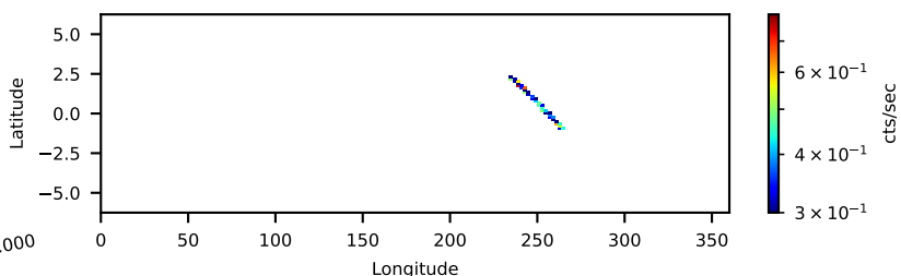
60965001001: 30 to 120 keV
