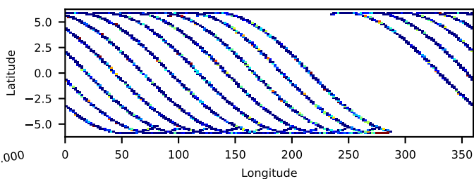
60964001002: 30 to 120 keV
