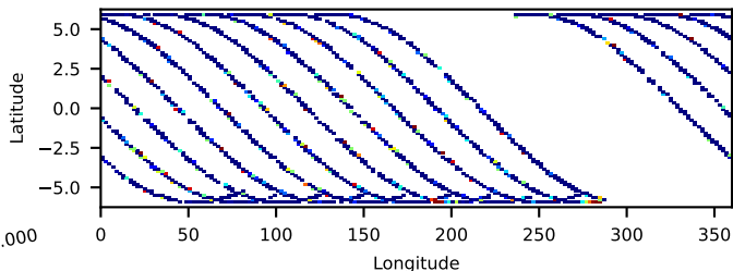
60964001002: 30 to 120 keV
