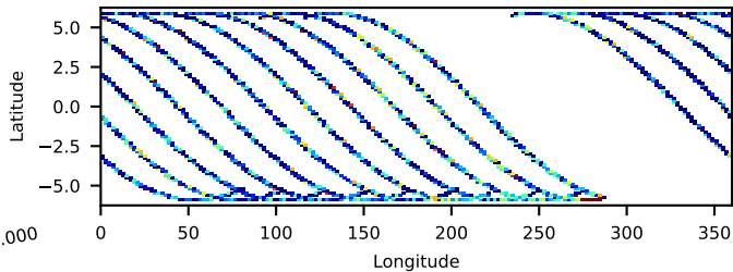
60964001002: 3 to 10 keV
