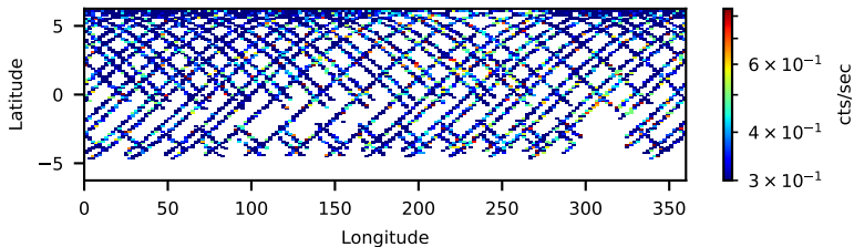
60963004002: 30 to 120 keV
