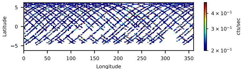
60963004002: 3 to 10 keV
