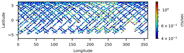
60963004002: 3 to 120 keV
