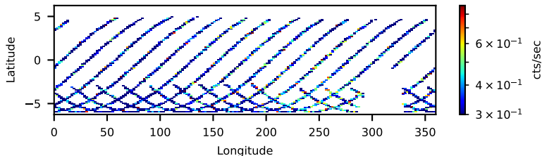
60962003002: 30 to 120 keV
