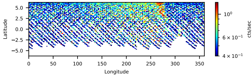
60961004002: 3 to 120 keV
