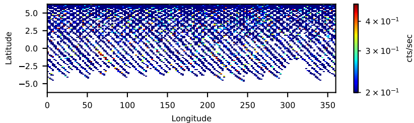
60961004002: 3 to 10 keV
