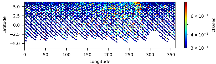
60961004002: 30 to 120 keV
