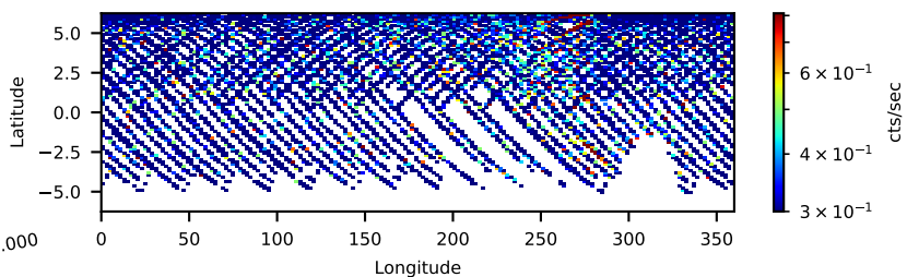
60961003002: 30 to 120 keV
