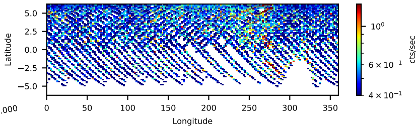
60961003002: 3 to 10 keV
