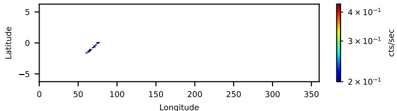
60961002001: 3 to 10 keV
