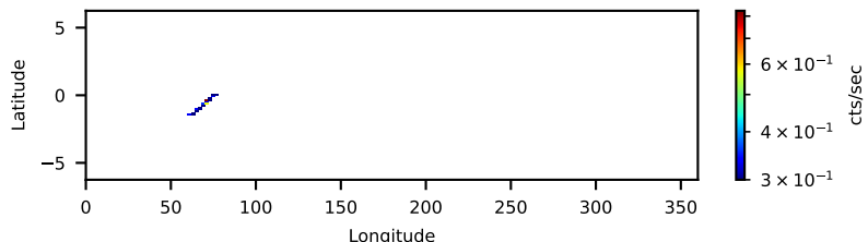
60961002001: 30 to 120 keV
