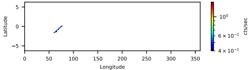
60961002001: 3 to 120 keV
