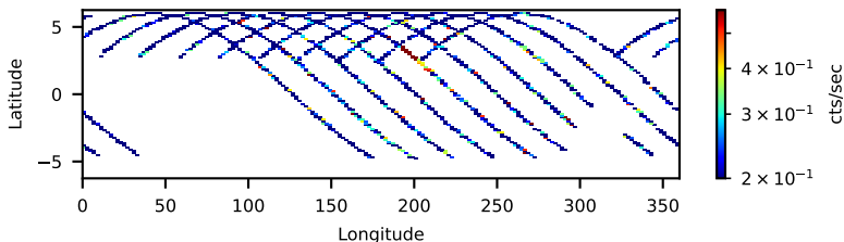
60960005002: 3 to 10 keV
