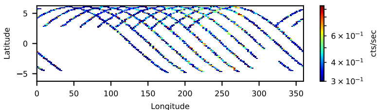
60960005002: 30 to 120 keV
