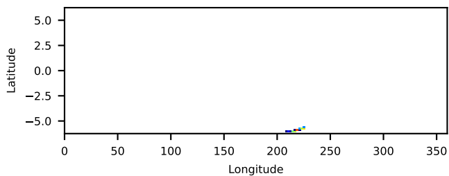
60960002001: 3 to 10 keV
