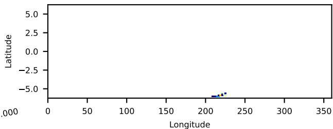
60960002001: 30 to 120 keV
