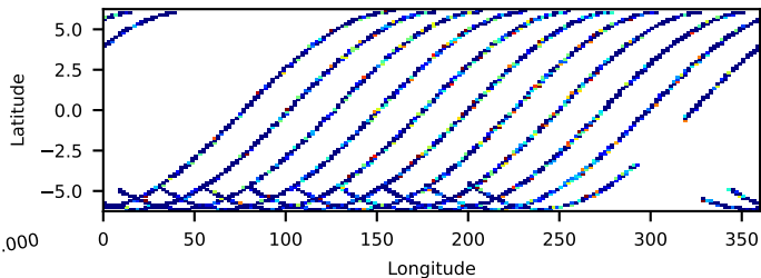
60902033002: 30 to 120 keV
