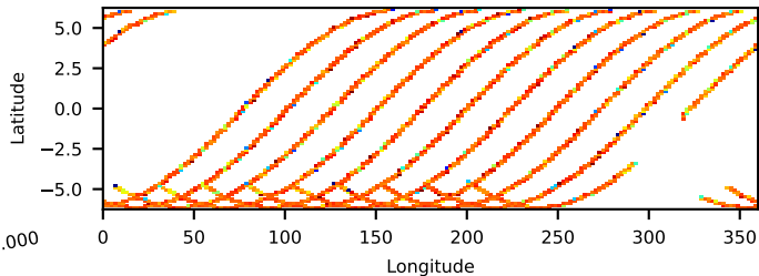
60902033002: 3 to 10 keV
