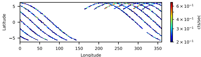
60902024012: 3 to 10 keV
