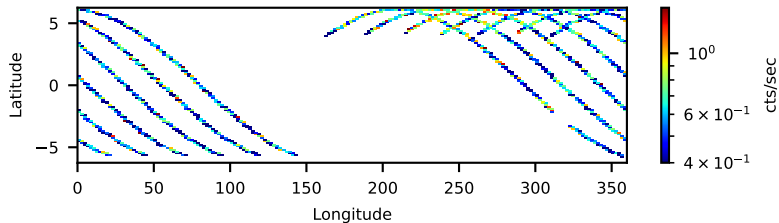
60902024012: 3 to 120 keV
