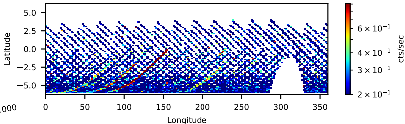
60902004002: 30 to 120 keV
