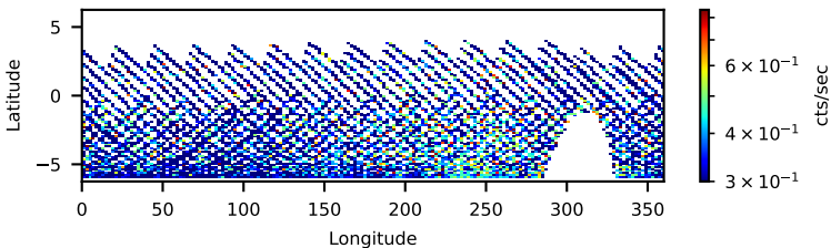
60902004002: 30 to 120 keV
