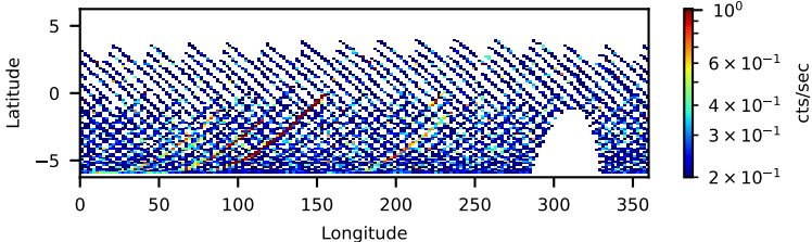
60902004002: 3 to 10 keV
