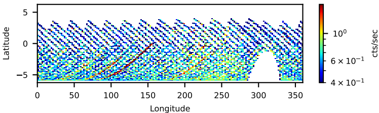
60902004002: 3 to 120 keV
