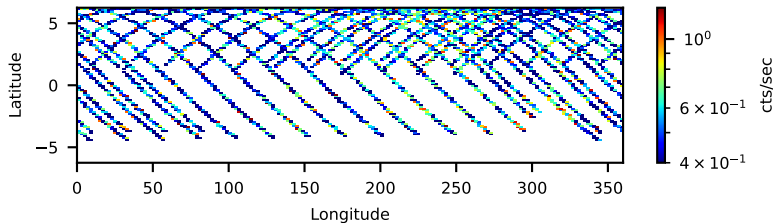
60902002002: 3 to 120 keV
