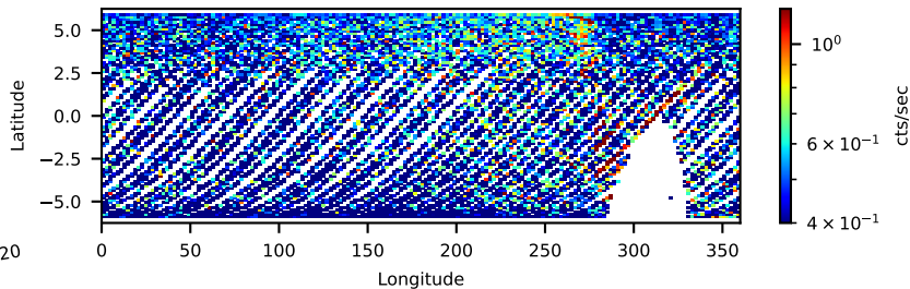
60901028002: 3 to 10 keV
