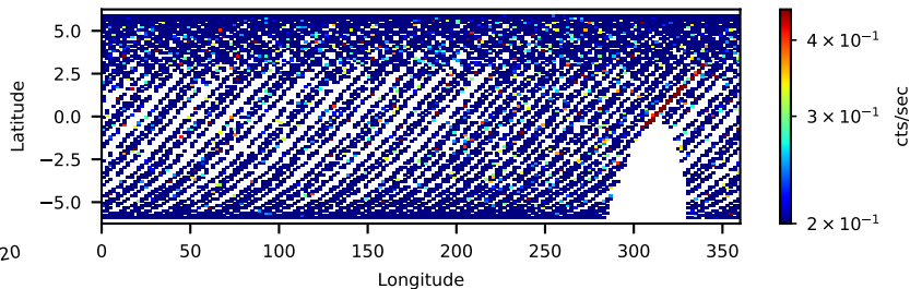
60901028002: 30 to 120 keV
