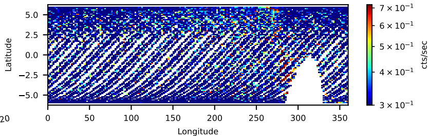
60901028002: 30 to 120 keV
