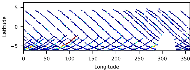
60901027002: 3 to 10 keV
