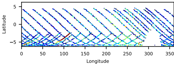
60901027002: 3 to 120 keV
