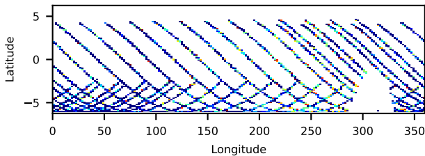
60901027002: 30 to 120 keV
