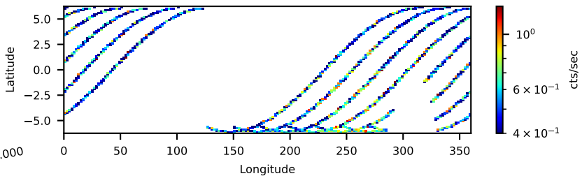
60901026002: 3 to 10 keV
