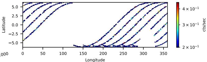
60901026002: 30 to 120 keV
