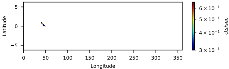
60901025001: 30 to 120 keV
