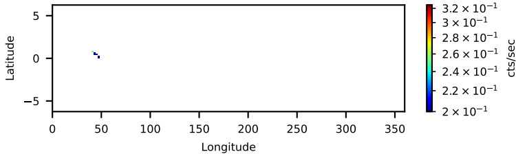
60901025001: 3 to 10 keV
