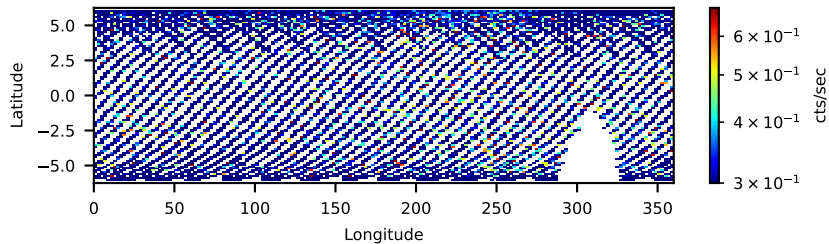
60901023002: 30 to 120 keV
