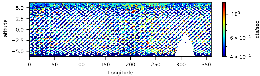
60901023002: 3 to 120 keV
