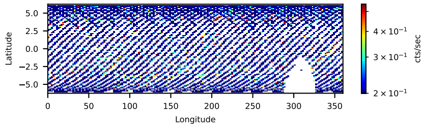
60901023002: 3 to 10 keV
