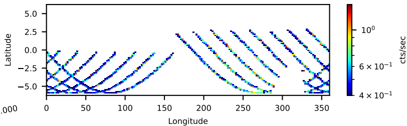
60901019002: 3 to 10 keV
