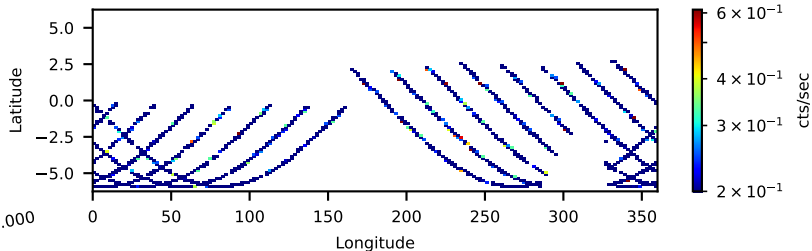
60901019002: 30 to 120 keV
