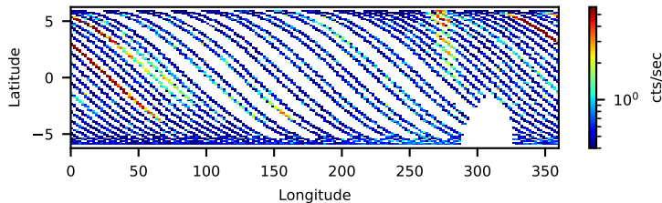
60901014004: 3 to 120 keV
