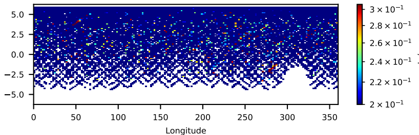
60901012002: 30 to 120 keV
