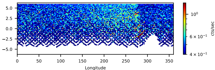
60901012002: 3 to 10 keV
