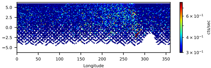
60901012002: 30 to 120 keV
