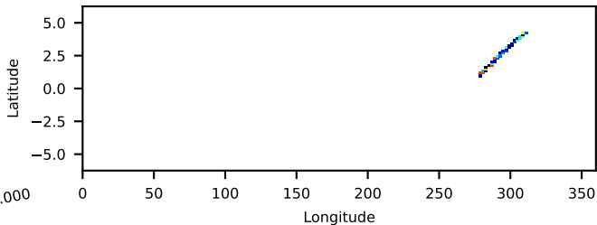
60864001001: 3 to 10 keV
