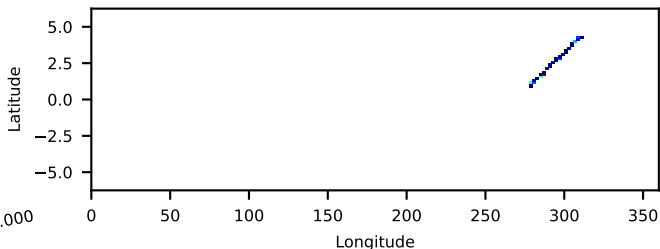
60864001001: 30 to 120 keV
