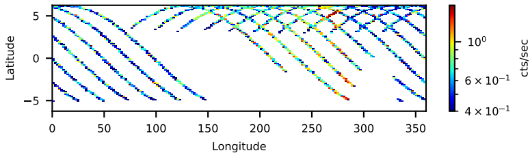
60863006002: 3 to 120 keV
