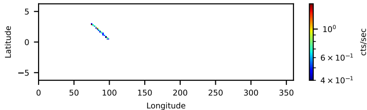
60863005001: 3 to 120 keV
