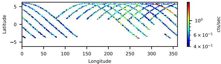
60863004002: 3 to 120 keV
