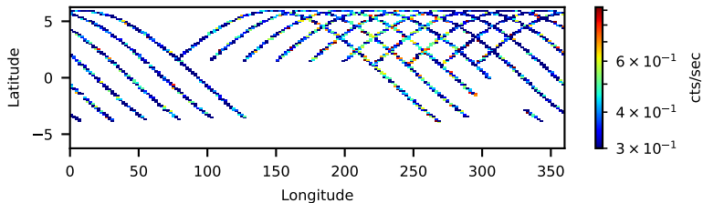
60863004002: 30 to 120 keV
