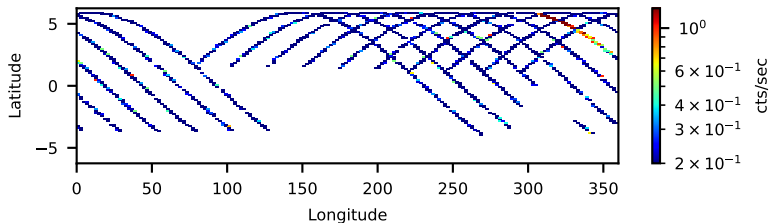
60863004002: 3 to 10 keV
