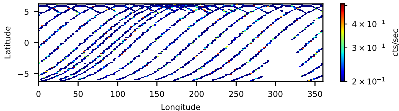
60862005002: 3 to 10 keV
