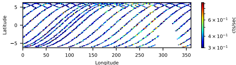
60862005002: 30 to 120 keV
