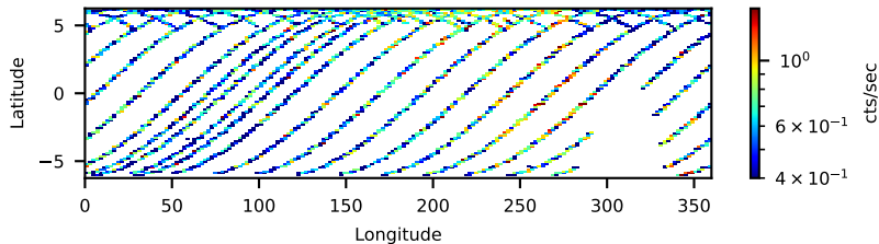
60862005002: 3 to 120 keV
