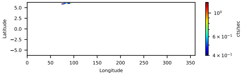
60862004001: 3 to 10 keV
