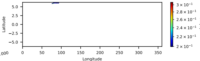
60862004001: 30 to 120 keV
