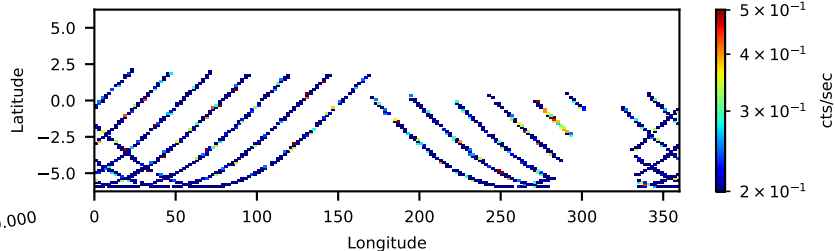
60862002002: 30 to 120 keV
