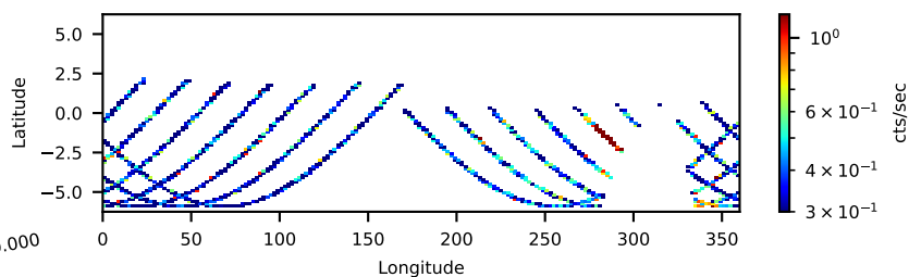
60862002002: 30 to 120 keV
