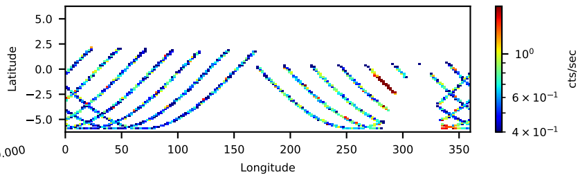
60862002002: 3 to 10 keV
